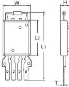
Dimension (尺寸图)
